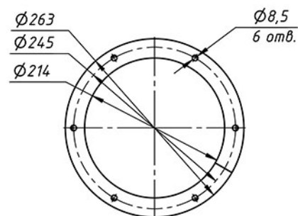
ВЫХОДНОЙ ФЛАНЕЦ
